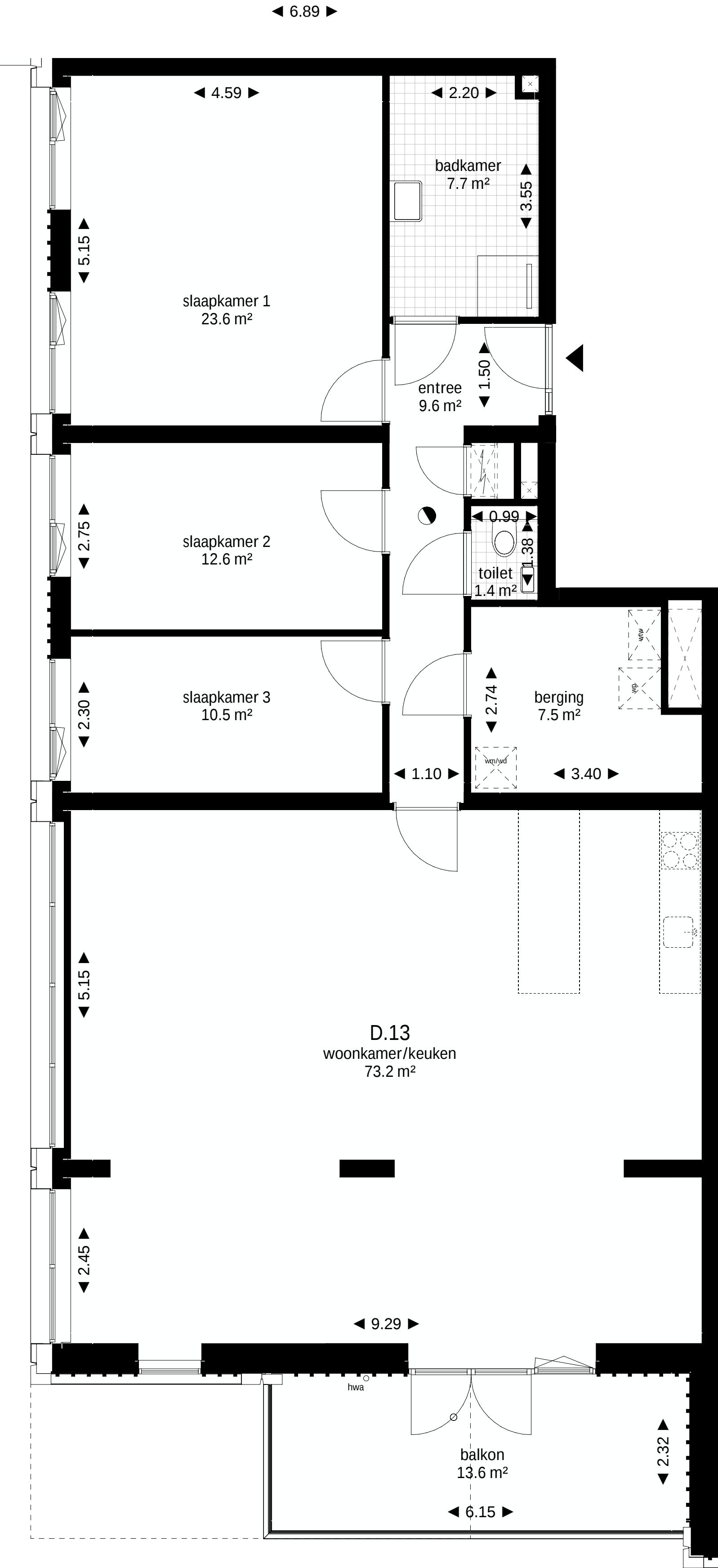
tweede verdieping 1 : 50
